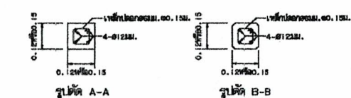
รูปตัดเลี้ยว
