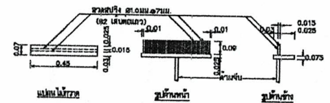
แบบขยายไม่หักเหล้าค.ส.ล.
