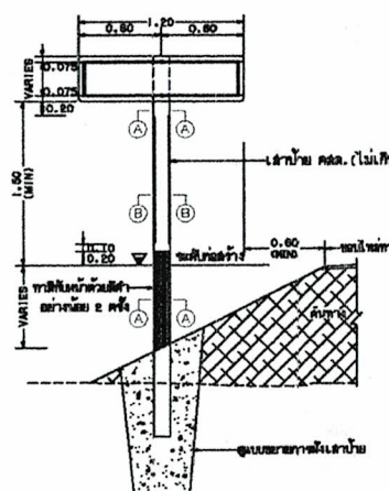
แสดงการติดตั้งป้ายแนะนำ น-1และน-4
