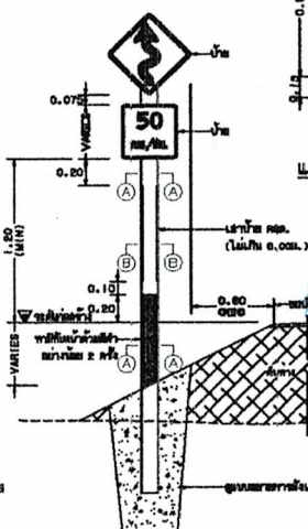
แสดงการติดตั้งป้ายบังคับและป้ายเตือน
