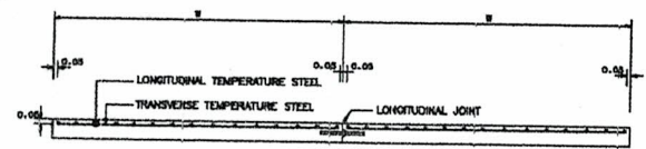
รูปตัดตามขวางเสริมเหล็ก ค.ส.ล.
