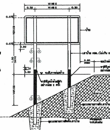
แสดงการติดตั้งป้ายแนะนำ น-2 น-3และน-5
