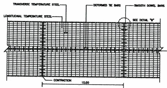
แบบขยายตามขวางเสริมเหล็ก ค.ส.ล.
