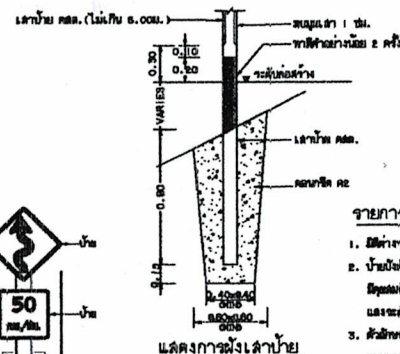
แสดงการติดตั้งป้าย
