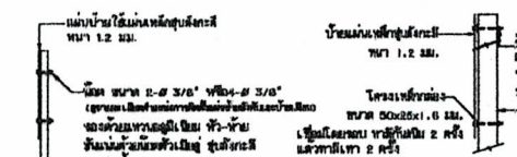
แสดงการติดตั้งป้ายบังคับป้ายเตือน
