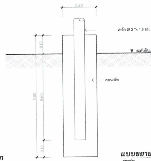
แบบแปลนขยายฐานราก มาตราส่วน 1:10
