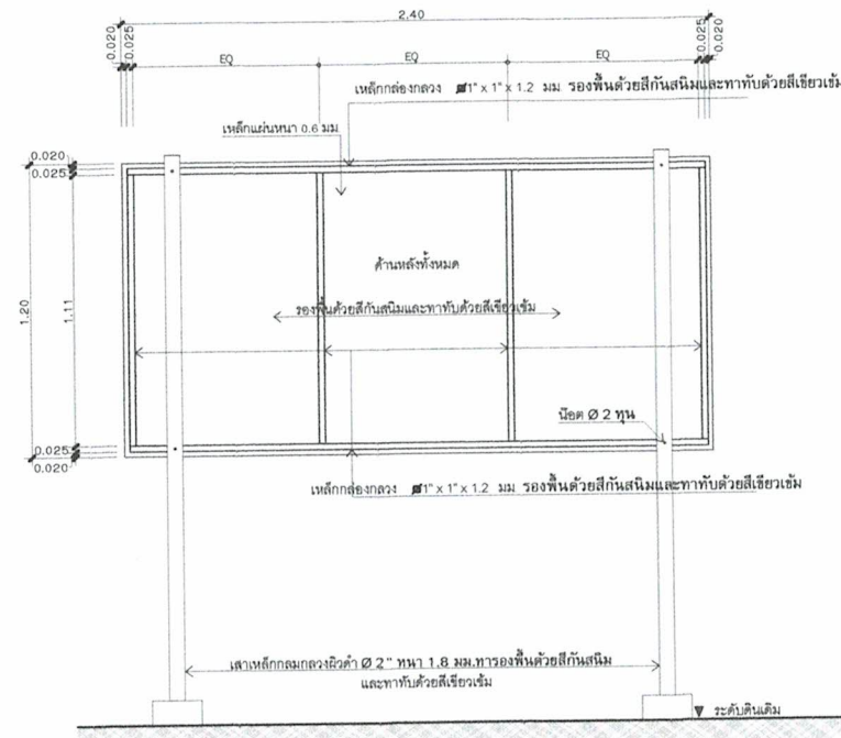
ด้านหลัง มาตราส่วน 1:25
